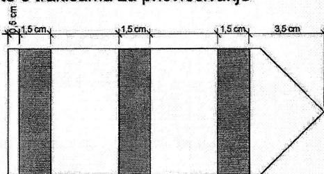
Skica 2. Donja strana epoleta s trakicama za pričvršćivanje
