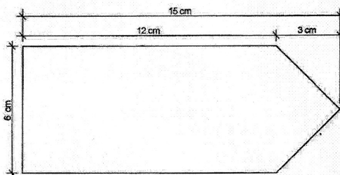
Skica 2. Donja strana epoleta s trakicama za pričvršćivanje
